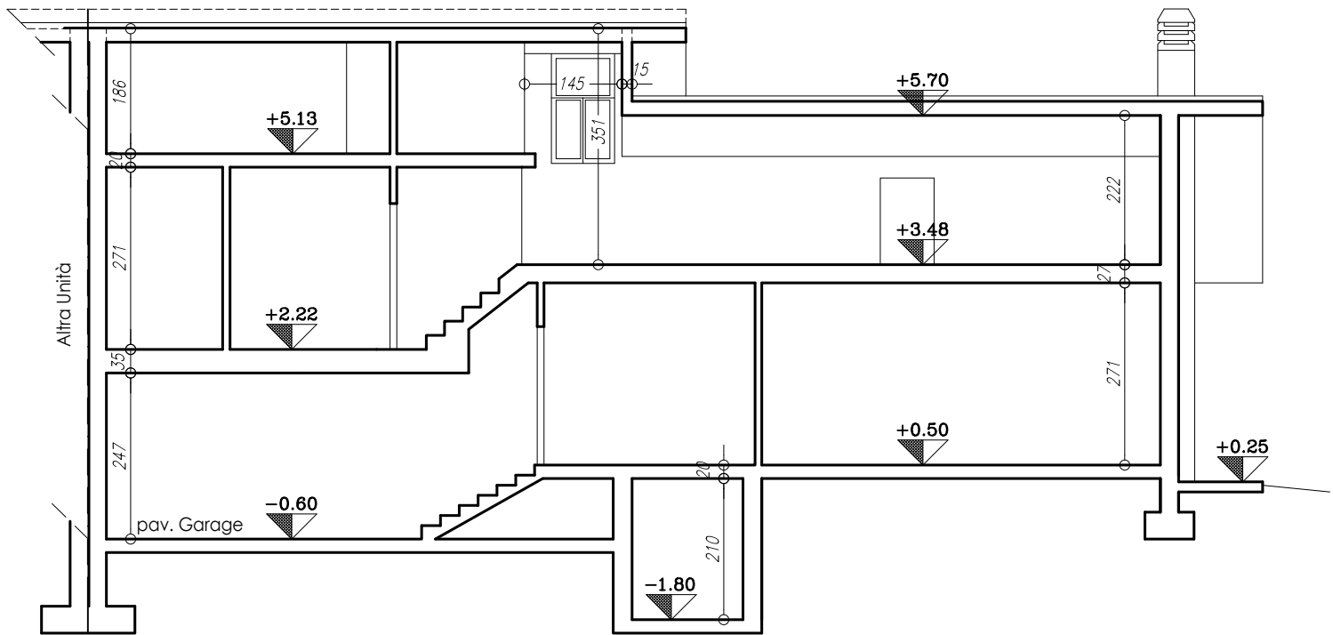
Sezione B-B
