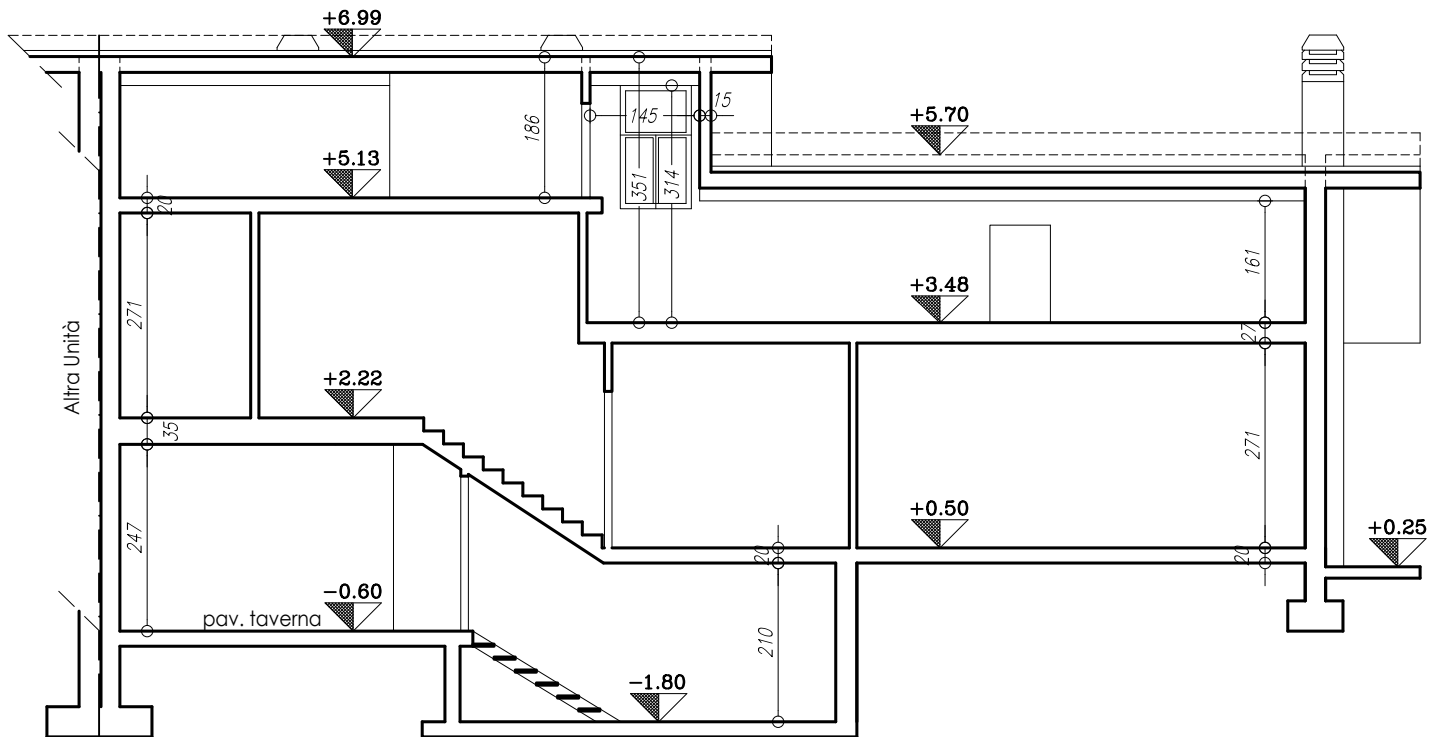
Sezione A-A
