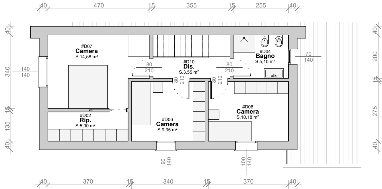
3 Pianta Piano Primo 1 : 100
