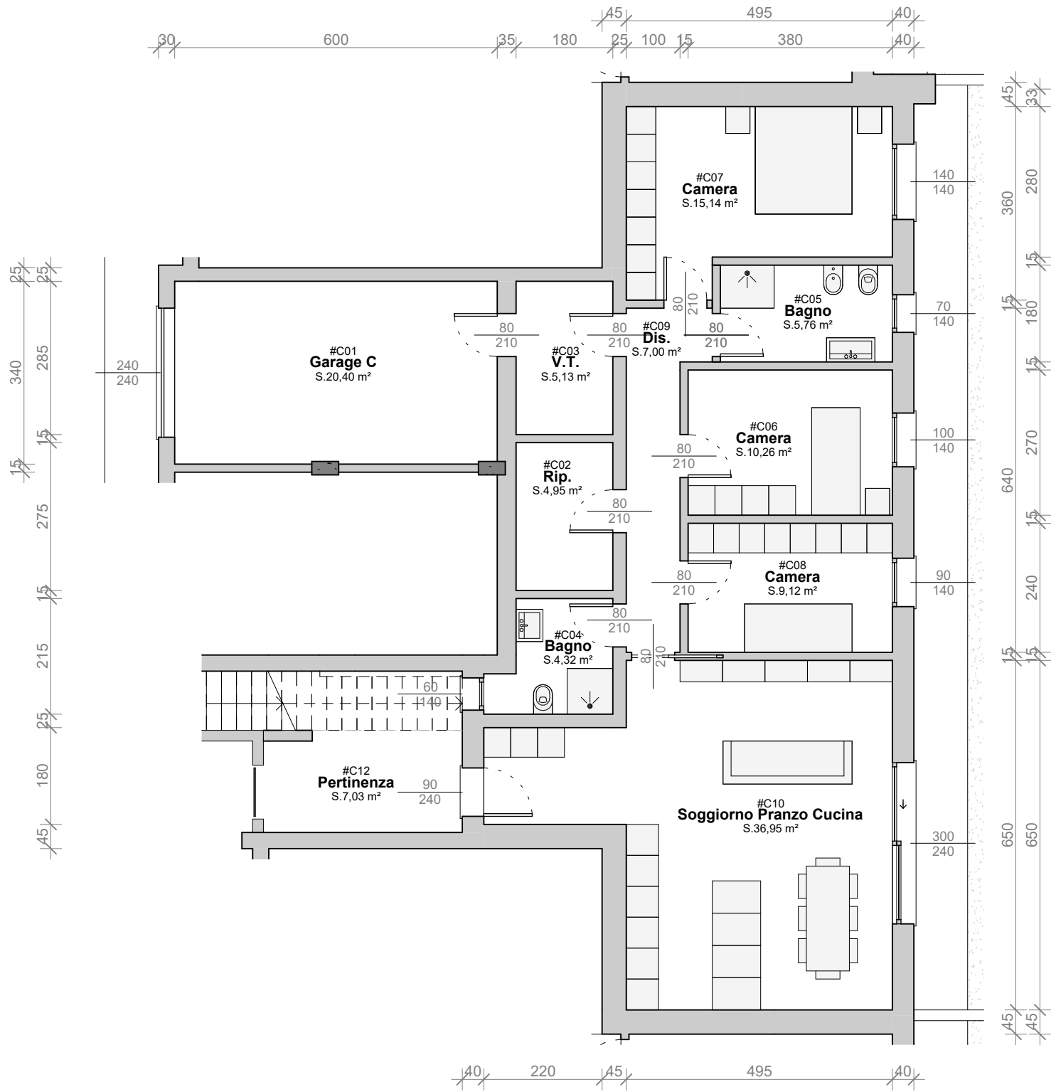
2 Pianta Piano Terra 1 : 100
