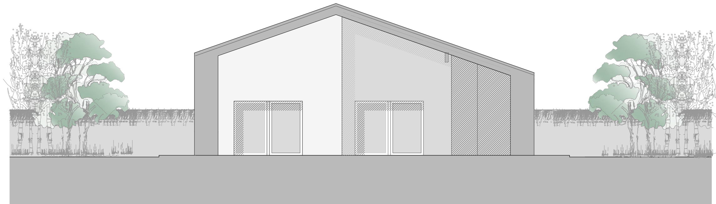
PROSPETTO OVEST - SC. 1:100
